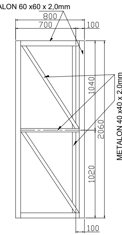
VISTA LATERAL
