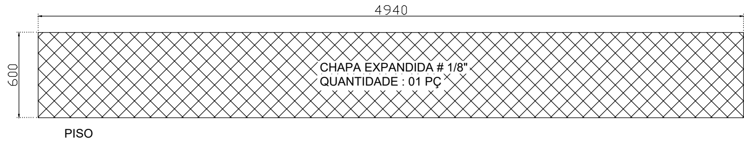
VISTA INFERIOR
