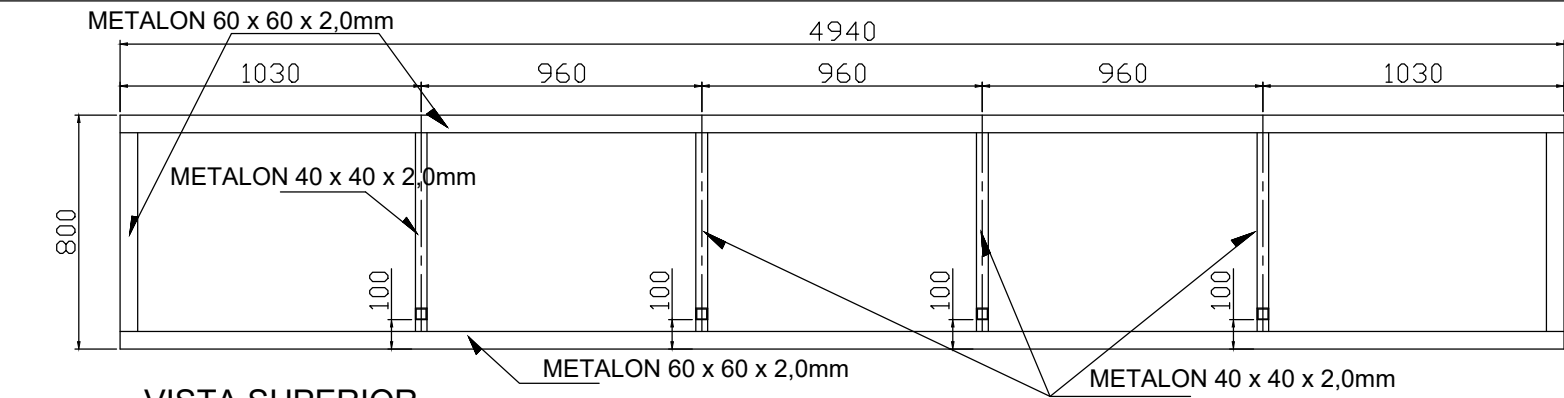
VISTA SUPERIOR
