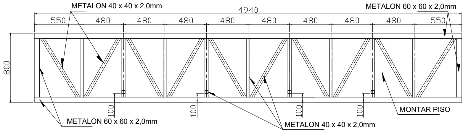
VISTA INFERIOR
